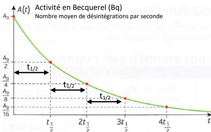
Courbe de décroissance radioactive
